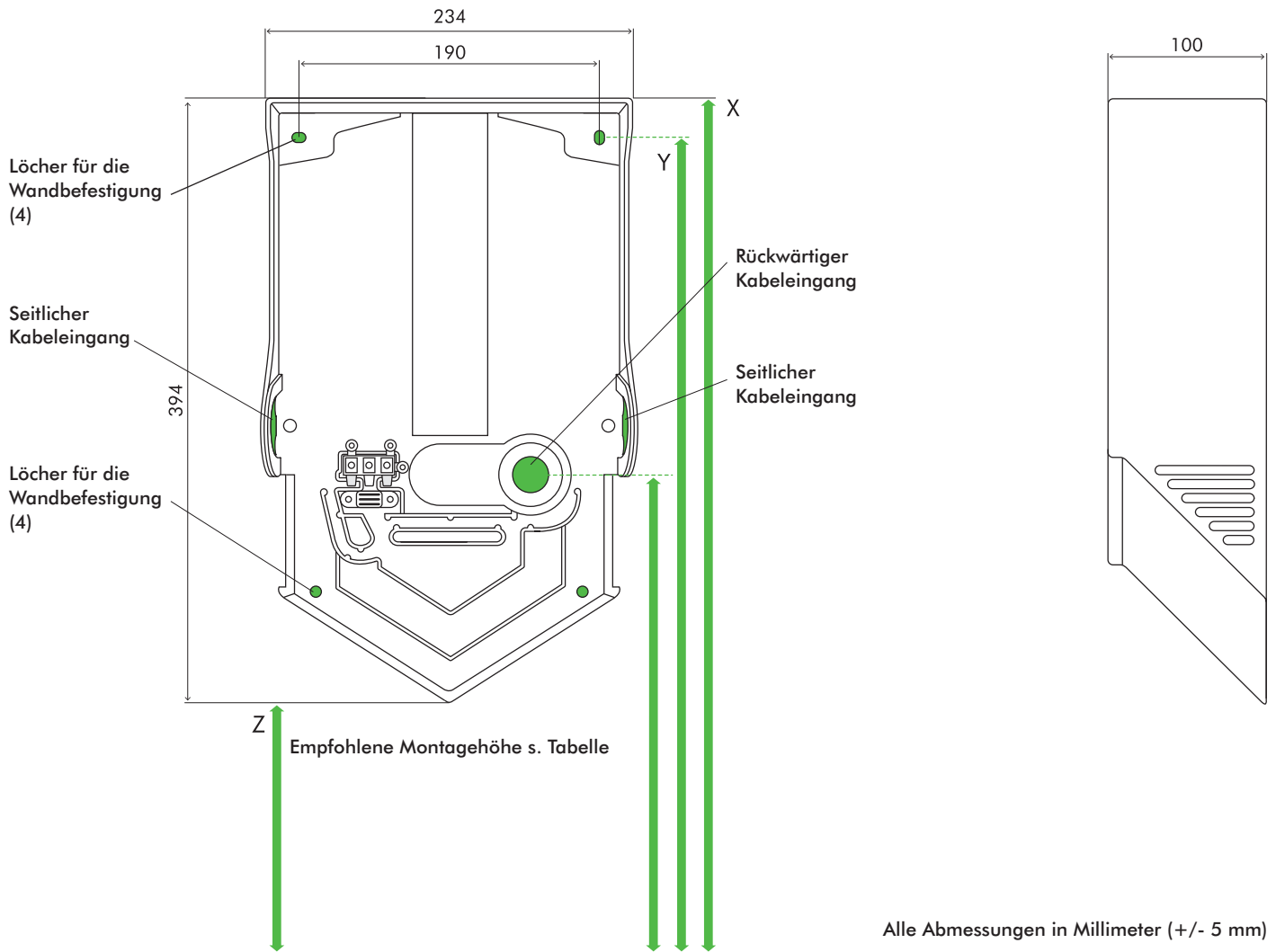
RÜCKANSICHT
